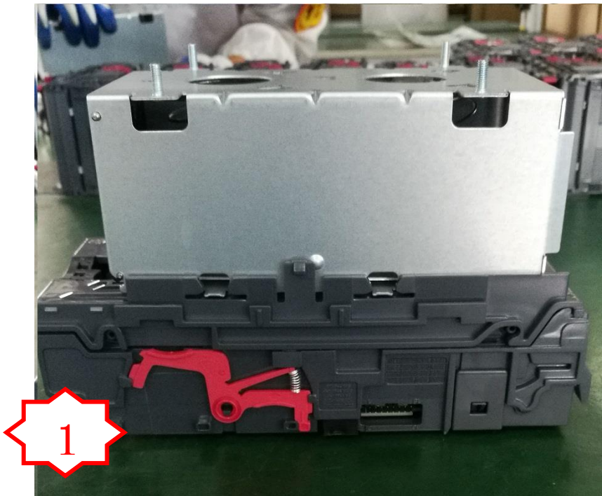
图一、将 PA898 如图放入 NV9ST 中，注意方向
