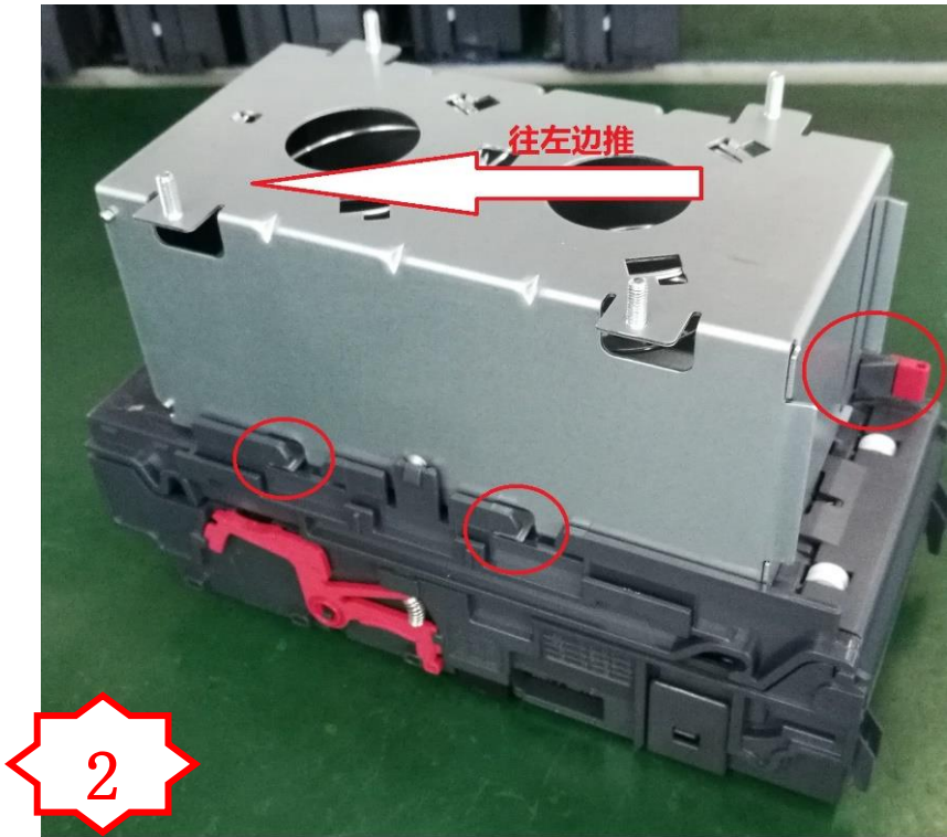
图二、往左推 PA898,注意装配到位，查看另外一边，也要装配到位
